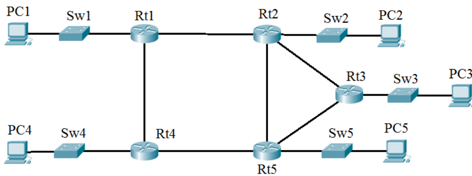
Рисунок 9 — Структурна схема віддаленого офісу №7
