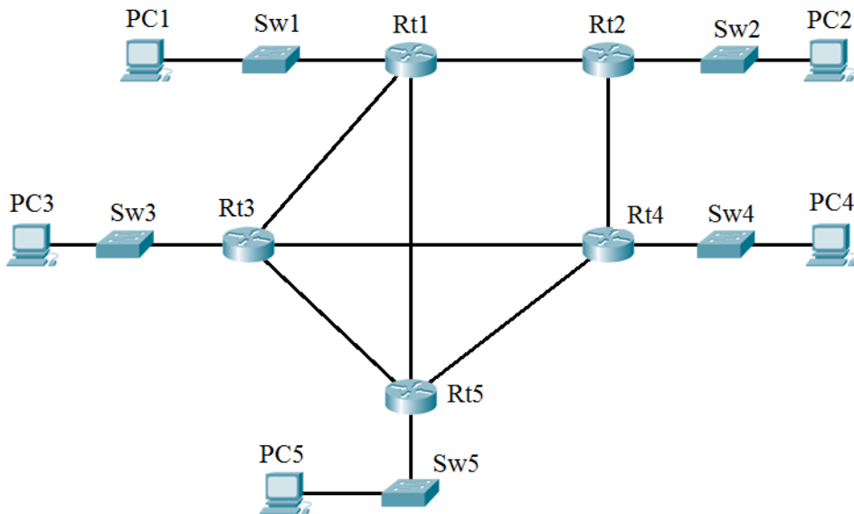
Рисунок 6 — Структурна схема віддаленого офісу №4
