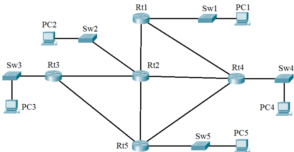
Рисунок 10 — Структурна схема віддаленого офісу №8
