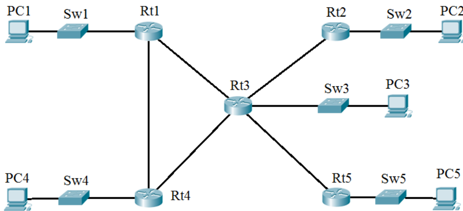
Рисунок 8 — Структурна схема віддаленого офісу №6
