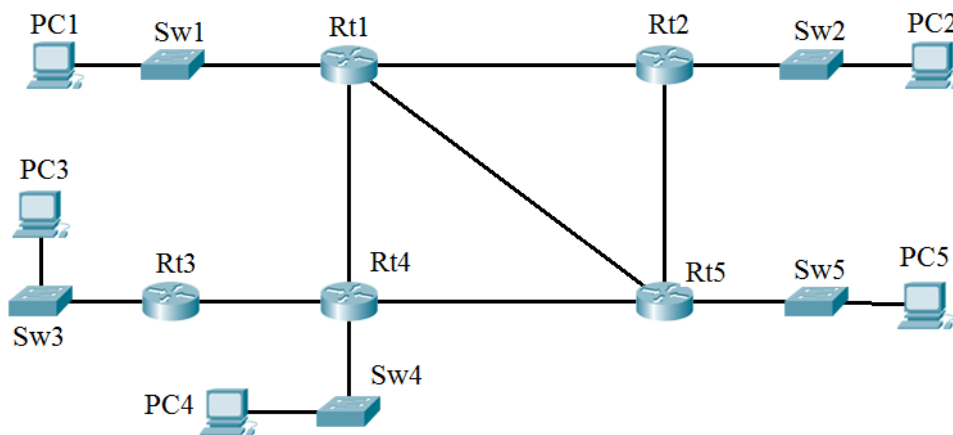
Рисунок 11 — Структурна схема віддаленого офісу №9
