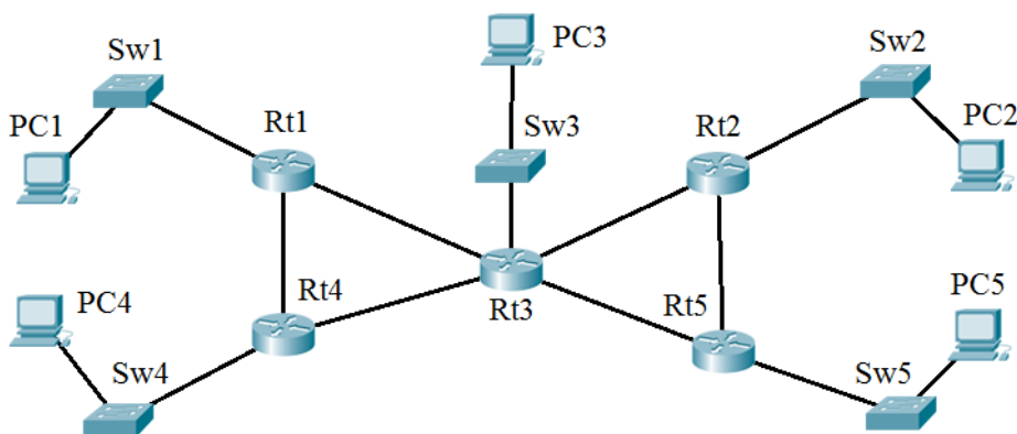
Рисунок 3 — Структурна схема віддаленого офісу №1
