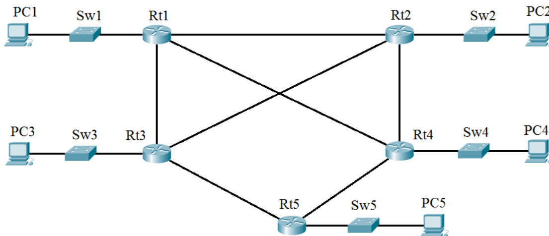
Рисунок 12 — Структурна схема віддаленого офісу №10
