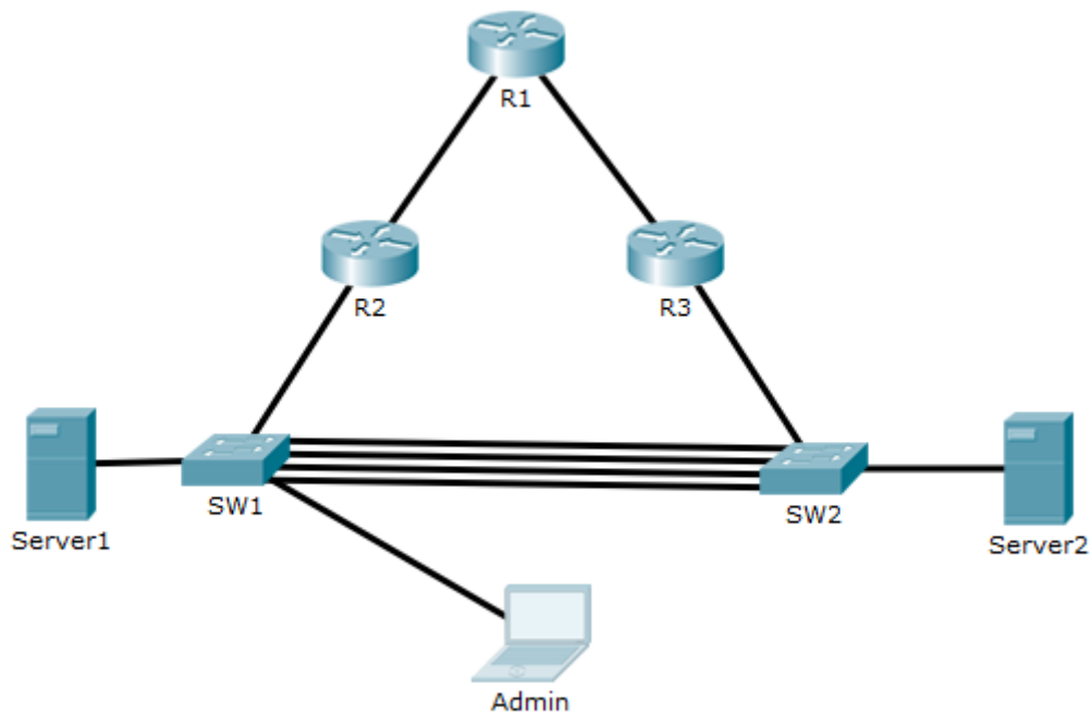
Рисунок 13 — Структурна схема дата центру
